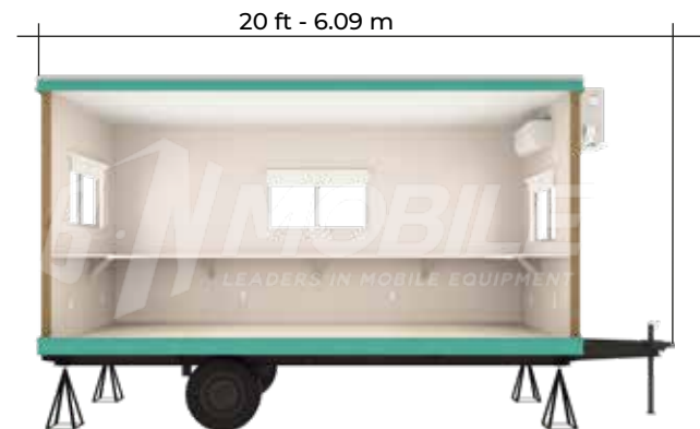
Corte
